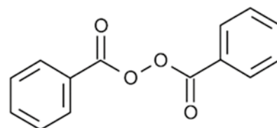
Obr. 1. Strukturní vzorec benzoylperoxidu (8)
